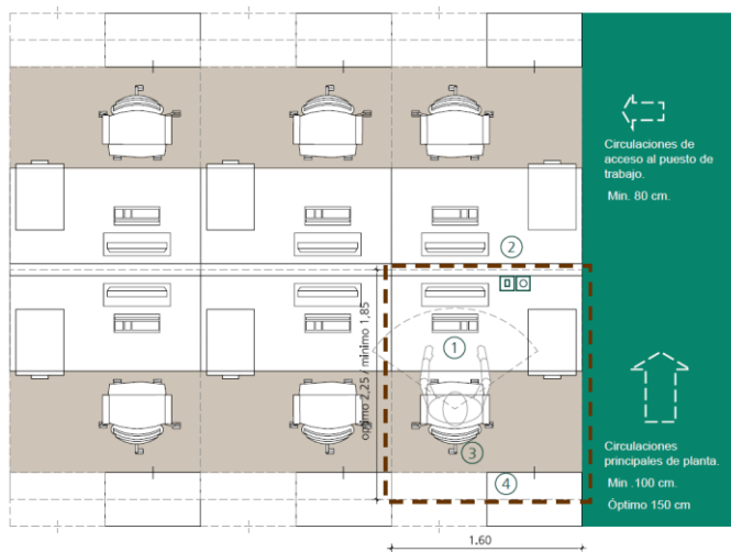
Gráfico 12. Puesto de trabajo tipo de en áreas abiertas para personal hasta nivel 21. Superficie sugerida: 3-4 m 2 . Fuente: UNED, op. cit. , p. 31.
