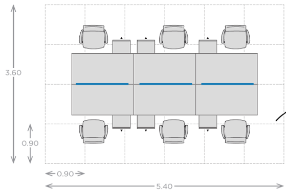
Gráfico 11. Modelo tipo de isla de trabajo en espacio abierto para 6 personas. Superficie sugerida: 3,25 m 2 por puesto. Fuente: Agencia de Administración de Bienes del Estado, op. cit. , p. 19.
