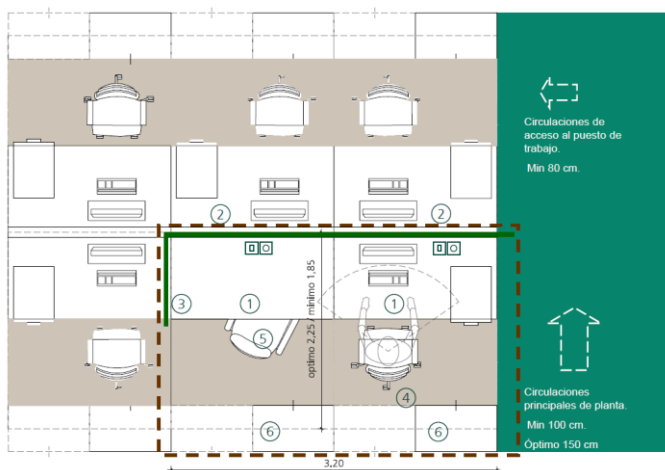
Gráfico 13. Modelo tipo de espacio de trabajo individual en áreas abiertas para personal de nivel 22 al 25. Superficie sugerida: 6-7 m 2 . Fuente: UNED, op. cit. , p. 31.
